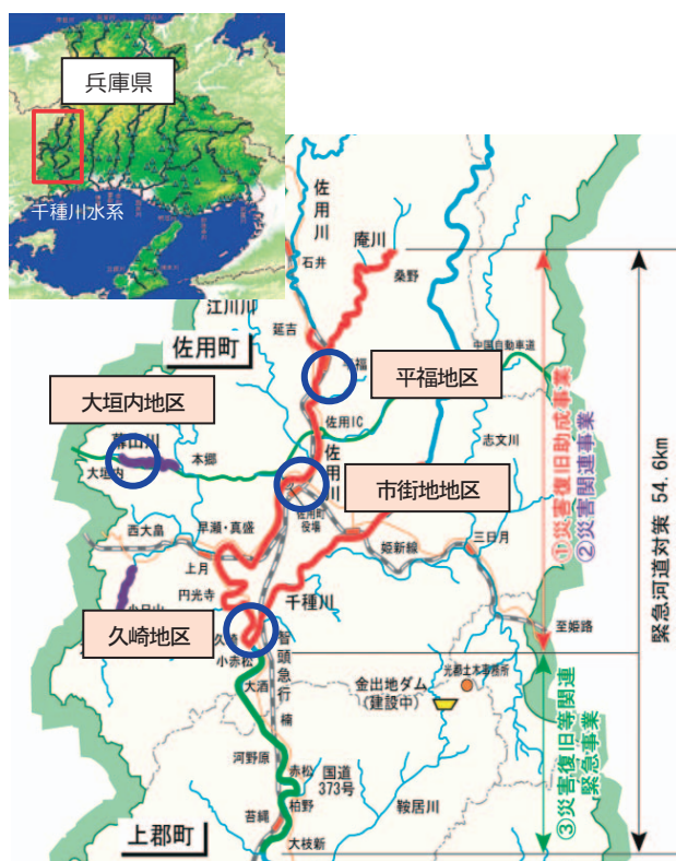
図－1 千種川水系緊急河道対策の概要
