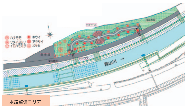
図-6 水路整備エリア概要図
