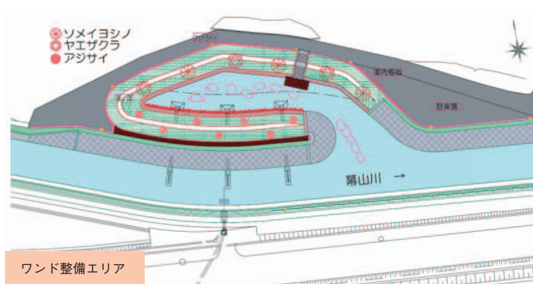
図-5 ワンド整備エリア概要図
